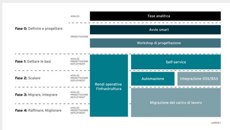
Figura 2. Schema dettagliato del Solution Delivery Framework di Red Hat Consulting
