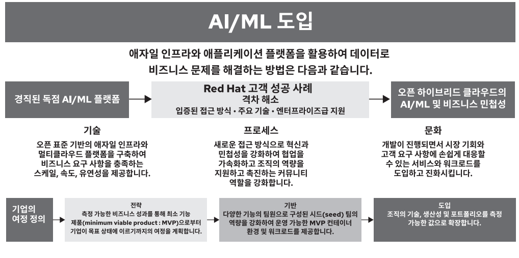
그림 1. AI/ML 도입
